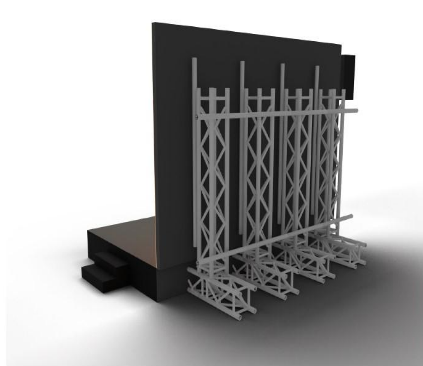
LED 4 m x 3,5 m struttura con T rovesciate
