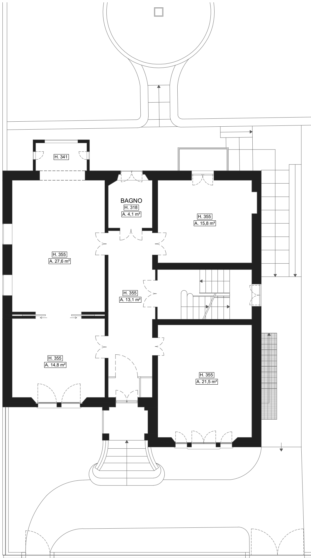
PIANTA PIANO RIALZATO 96,7 m 2 - Scala 1:100
