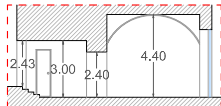
Sezione D-D'
