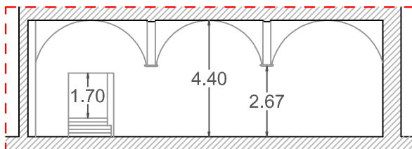
Sezione C-C'
