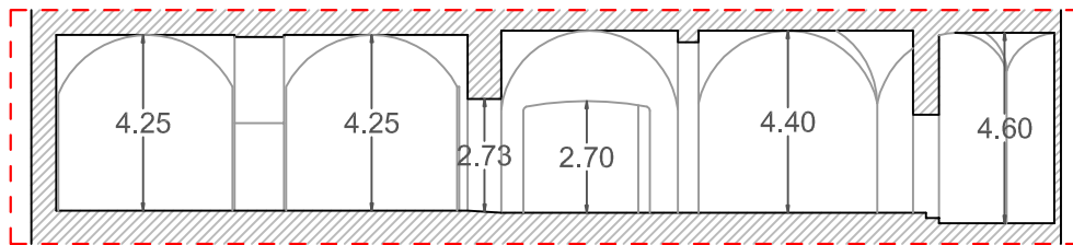
Sezione B-B'
