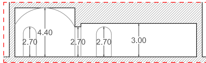
Sezione A-A'
