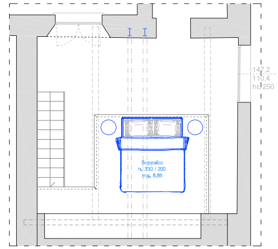
SOPPALCO - Appartamento 1
