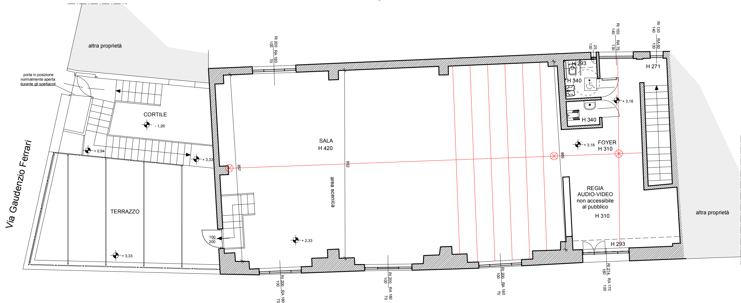
PLANIMETRIA PIANO PRIMO
